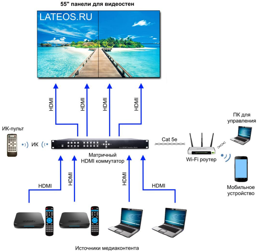
Рис. 3 Схема построения видеостены на базе матричного HDMI коммутатора
